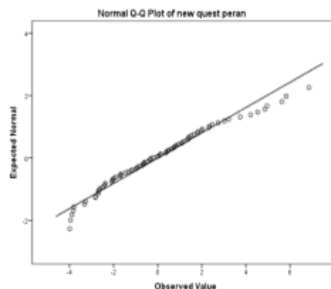
Gambar 3.3 Q – Q Plot Uji Normalitas Peran Orang Tua
