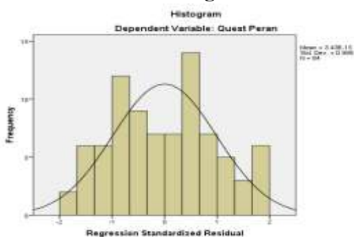
Gambar 3.2 Histogram Uji Normalitas Peran Orang Tua
